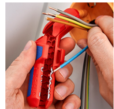
Удаление изоляции с отдельных проводов
